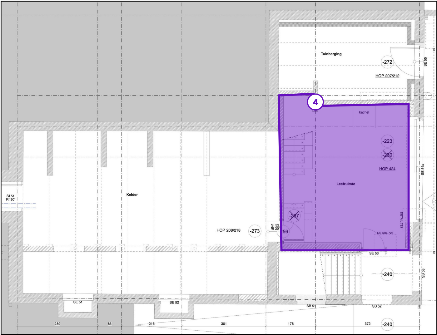
Legende van plan 1.1: Plan woning -1 en kelder
