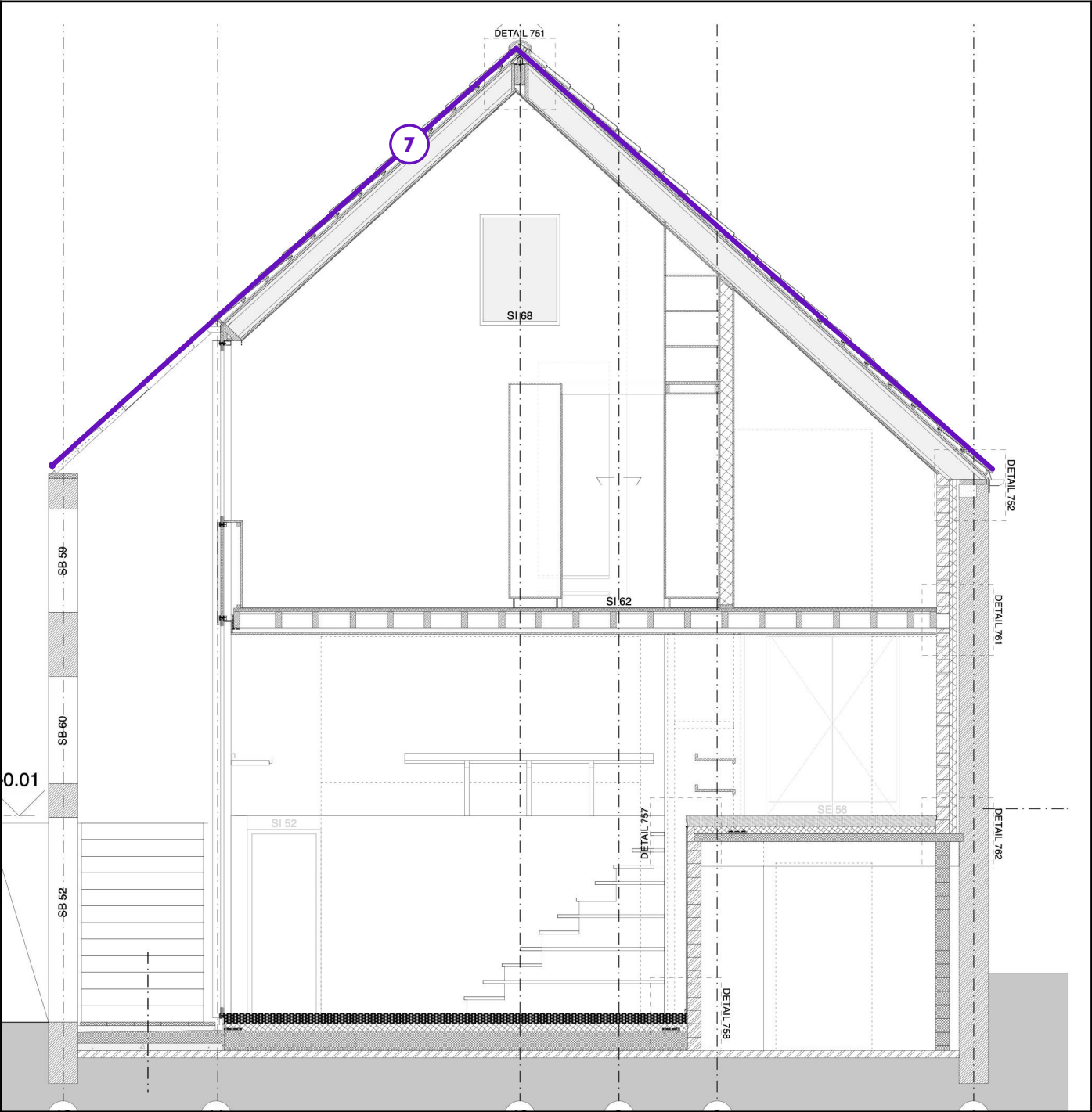
Legende van plan 1.14: Doorsnede woning
