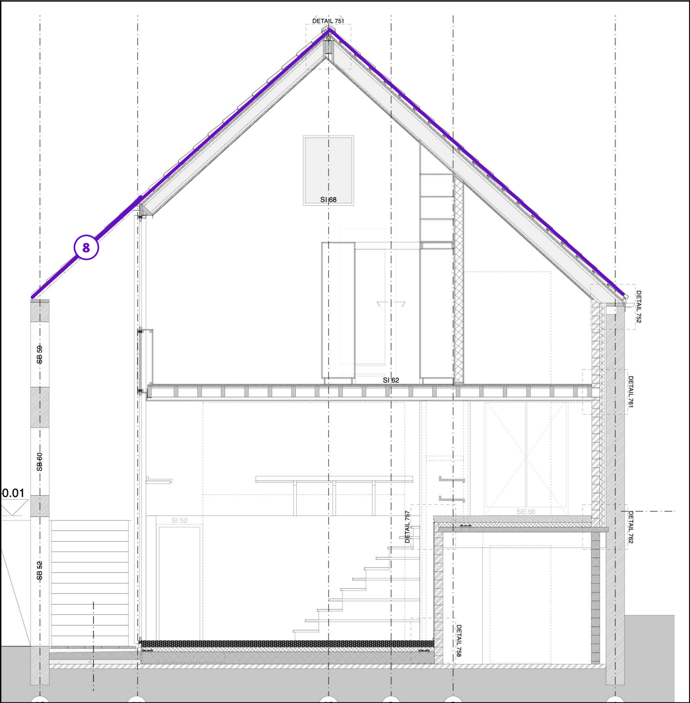
Legende van plan 1.7: Doorsnede woning
